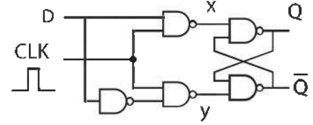
চিত্র 3.22 : DQ ফ্লিপফ্লপ-এর ভিত্তরীণ গঠন
