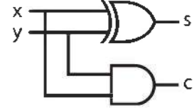
চিত্র 3.18 : x এবং y এই দুইটি বিট যোগ করার জন্য হাফ এডারের সত্যক সারণি এবং এই সত্যক সারণি বাস্তবায়নের জন্য প্রয়োজনীয় সার্কিট
