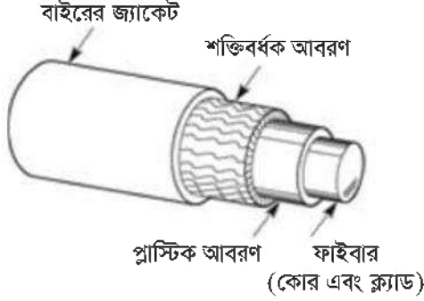
চিত্র ২.৯: অপটিক্যাল ফাইবারের গঠন
