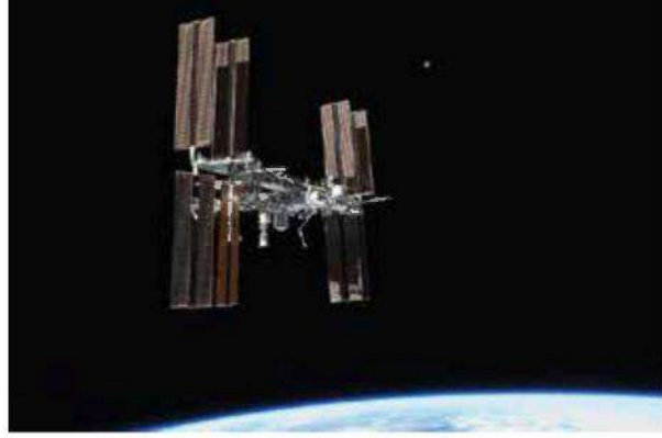
চিত্র 1.11 : পৃথিবীকে ঘিরে ঘূর্ণায়মান মহাকাশ স্টেশন
