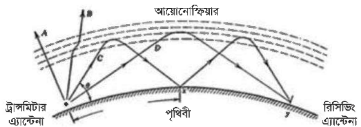
চিত্র 2.12: পৃথিবী গুঁঠে রেডিও ওয়েভের ট্রানমিশন
