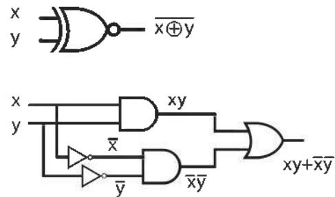
চিত্র 3.13 : X-NOR গেটের সত্যক সারণী, প্রতীক এবং লজিক
