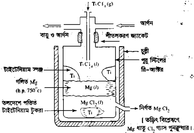
চিত্র ৩.৭ : টাইটেনিয়াম ধাতু নিষ্কাশন।
