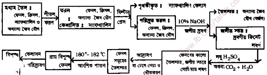
চিত্র ৭.৭ : মধ্যম তৈল থেকে বিশুদ্ধ ফেনল নিষ্কাশন এর প্রবাহচিত্র
