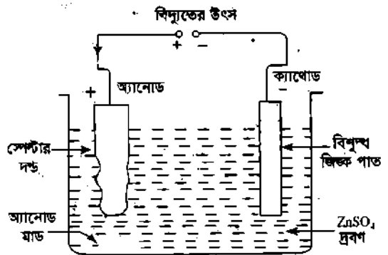
চিত্র ৩.১৭ : অবিশুদ্ধ জিংকে বা স্পেল্টারের বিদ্যুৎ বিশুদ্ধিকরণ।
