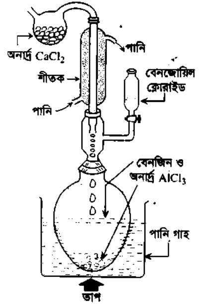
চিত্র ৮.৬ : পরীক্ষাগারে বেনজোফেনোন প্রস্তুতি।
