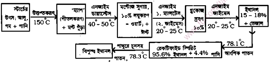
চিত্র ৭.৩ : স্টার্চ থেকে বিশুদ্ধ ইথানল উৎপাদনের প্রবাহচিত্র
