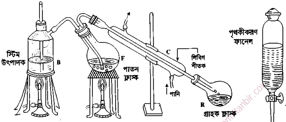
চিত্র ১২.৮ : বাষ্প পাতন পদ্ধতি।
