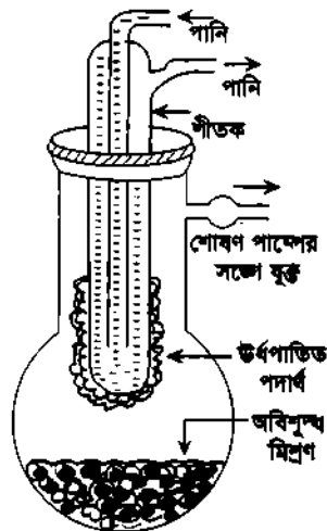
চিত্র ১২.৫ : নির চাপে উর্ধ্বপাতন।
