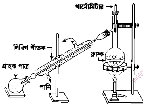
চিত্র ১২.৬ : পাতন পদ্ধতি।
