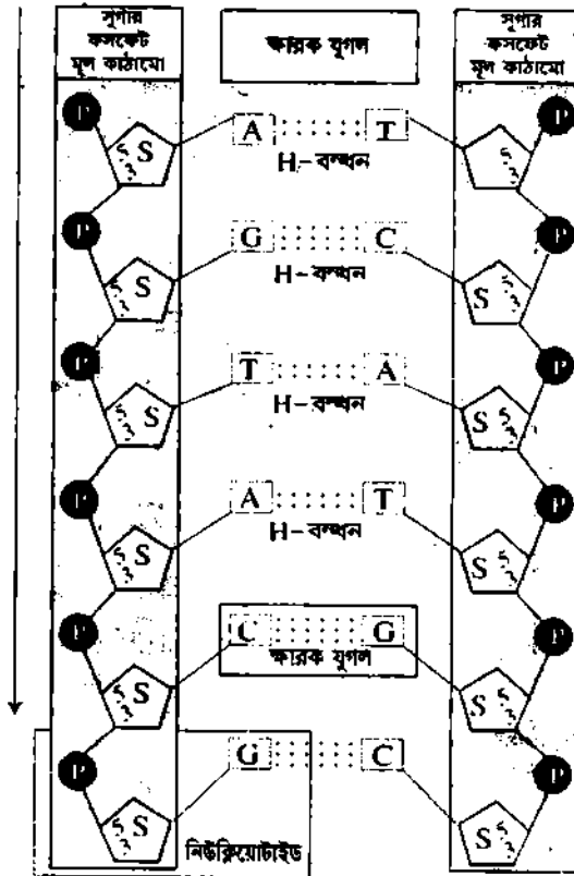
চিত্র ১১.২৪ : DNA এর রাসায়নিক স্ট্রিকচার।
