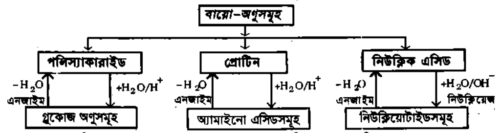
চিত্র ১১.২ : বায়ো-অণুসমূহের মনোমার ও পলিমারের পারস্পরিক রূপান্তর
