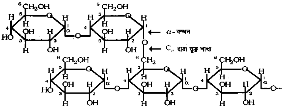
চিত্র ১১.১০ : শাখাবদ্ধ অ্যামাইলো-পেকটিন শিকল।
