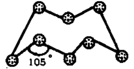
চিত্র ১.১৯ : মুকুট আকৃতির \text{S}_8 অণু গঠন
