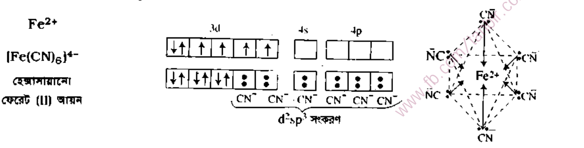
চিত্র ৩.৪ : [Fe(CN)_6]^{4-} আয়নের অষ্টতলকীয় গঠন।
