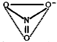
চিত্র ১.২৮ : নাইট্রেট আয়নের গঠন।
