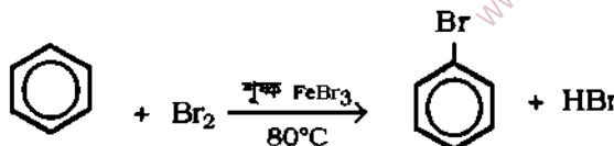
ব্রোমো বেনজিন
