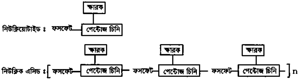
চিত্র ১১.১৯ : নিউক্লিয়োটাইড ও নিউক্লিক এসিডের আকরিক গঠন।
