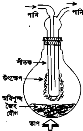
চিত্র ১২.৪ : উর্ধ্বপাতন।
