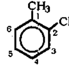
2-ক্লোরো টলুইন
