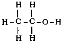
ইথানল অ্যালকোহল বা ইথানল
