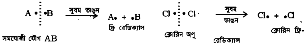
চিত্র ৪.১১ : সমযোজী সিগমা বন্ধনের সুষম ভাঙন।
