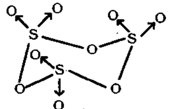
চিত্র ১.২৪ : কঠিন অবস্থায় ট্রাইমার (SO 3 ) 3
