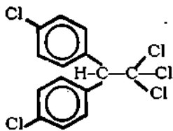
D. D. T.
