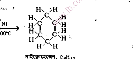
সাইক্লোহেক্সেন, \text{C}_6\text{H}_{12}
