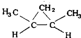
সিস্ - 1,2-ডাইমিথাইল সাইক্লোপ্রোপেন
