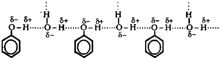
চিত্র ৭.৯ : পানি অণু ও ফেনল অণুর মধ্যে হাইড্রোজেন বন্ধন (ডট চিহ্ন ..... দ্বারা দেখানো হল)
