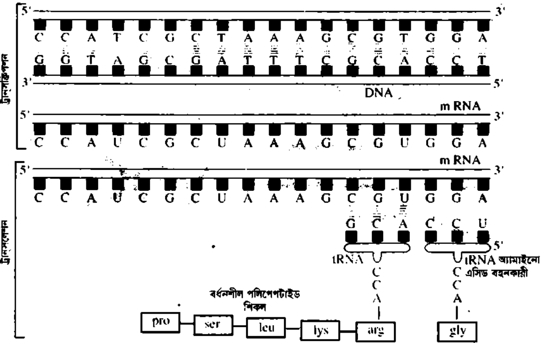
চিত্র ১১.২৮ : (ক) ট্রান্সক্রিপশন : DNA শিকলের সম্পূর্ণ mRNA গঠন : (খ) ট্রান্সলেশন : mRNA শিকায়ের (কোডন) এর সাথে সম্পূর্ণ tRNA (অ্যাকটিকোডন)
