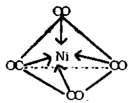
চিত্র ৩.৪(ক) : Ni(CO)_4 অণুর চতুষ্তলকীয় গঠন।
