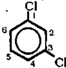
1, 3.-ডাইক্লোরো বেনজিন
