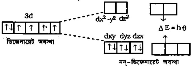
চিত্র ৩.৫ : লিগ্যান্ডের আপমানে d-অরবিটালসমূহের দুটি পৃথক শক্তিস্তরে বিন্যস্তকরণ।
