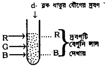
Green (সবুজ বর্ণ) এর শোষণ ঘটে।
