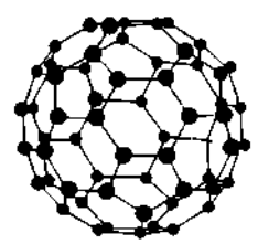
চিত্র ৪.১ : ফুলারিন
