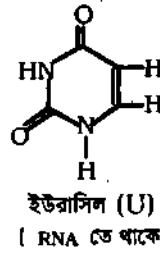
চিত্র ১১.১৭ঃ পিরিমিডিন কারকসমূহ।
