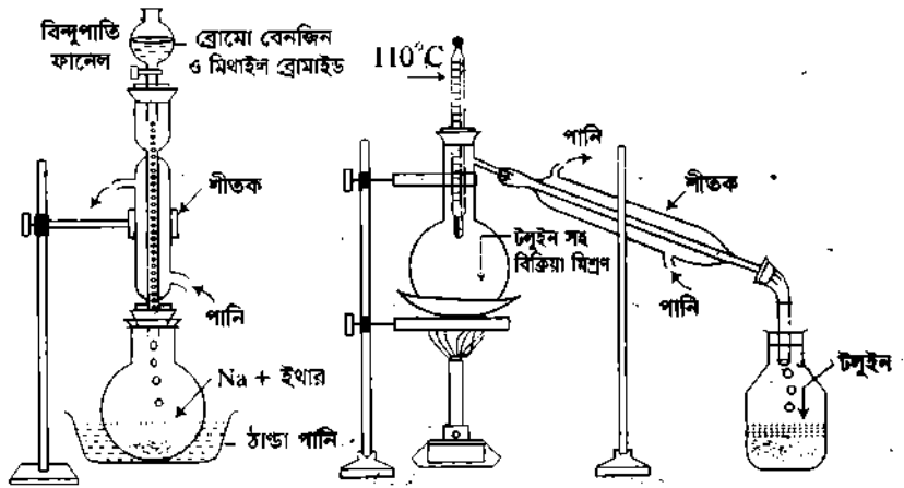
চিত্র ৫.৭ : পরীক্ষাগারে টলুইন প্রস্তুতি।
