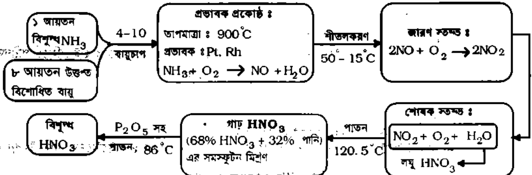
চিত্র ১.১২.১ অসওয়াল্ড প্রণালীতে অ্যামোনিয়া থেকে নাইট্রিক এসিড উৎপাদনের প্রবাহ চিত্র।
