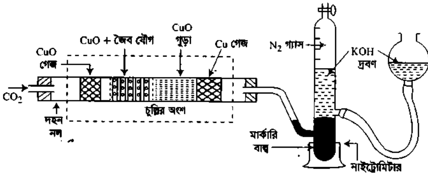
চিত্র-১২.২০ : ডুমার পদ্ধতিতে N-এর পরিমাণ নির্ণয়
