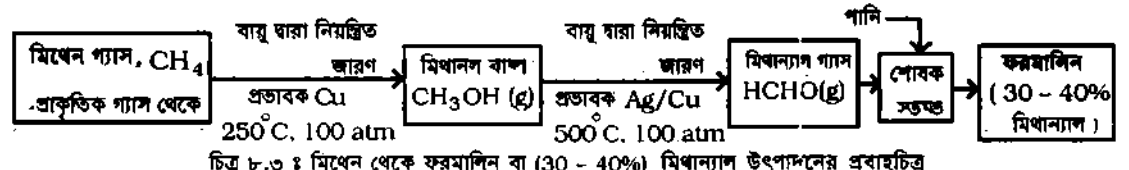
চিত্র ৮.৩ : মিথেন থেকে ফরমালিন বা (30 - 40%) মিথান্যাল উৎপাদনের প্রবাহচিত্র
