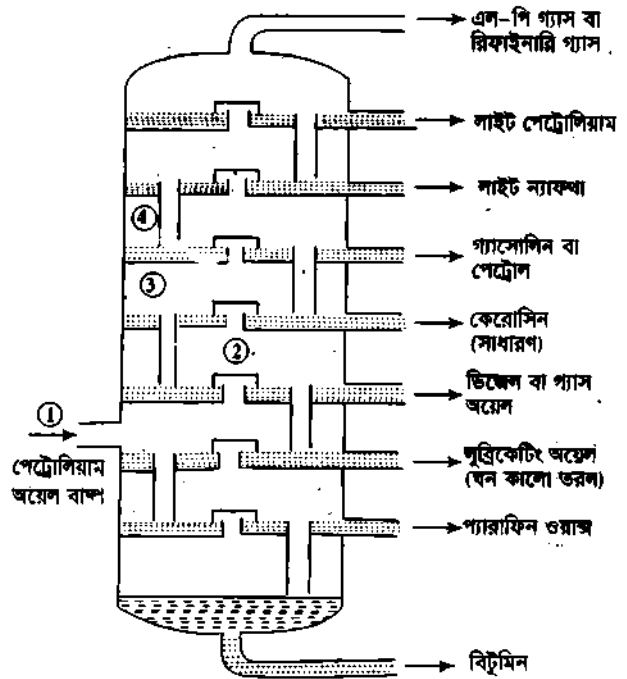
চিত্র ৫.১ : অপোখিত বা কুড পেট্রোলিয়ামের আংশিক পাতন।
