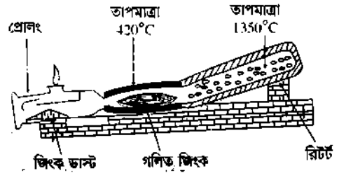
চিত্র ৩.১৬ : জিংকে অক্সাইডের বিজারণ।
