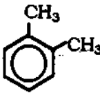
অর্ধে ডাইমিথাইল বেনজিন বা, o -জাইলিন
