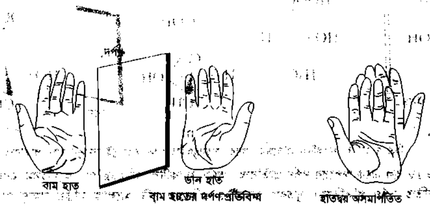
চিত্র ৪.১৯ : ডান হাত বাম হাতের দর্পণ প্রতিবিম্ব এবং হাতদ্বয় অসমাপতিত।
