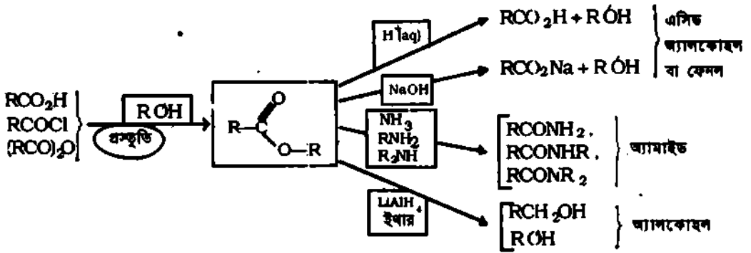
চিত্র ৯.৮ : বিভিন্ন পদ্ধতিতে এস্টার প্রস্তুতি ও এস্টারের বিক্রিয়ার চিত্রসূত্র
