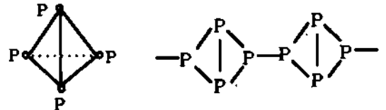
শ্বেত ফসফরাস এর P_4 অণুর গঠন;
