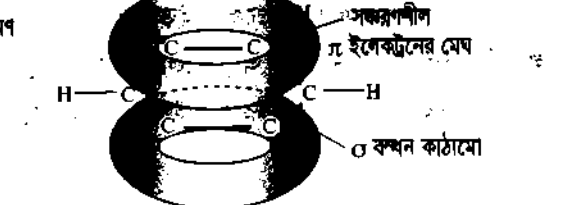
চিত্র ৫.৯ : মাঝখানের ছয় কার্বনের ষড়ভুজাকার সমতলটি \sigma বন্ধন দ্বারা সৃষ্ট। ওপরে ও নিচে p অরবিটালের পাশাপাশি অধিক্রমণ।
