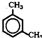
মেটা ডাইমিথাইল বেনজিন বা, m -জাইলিন
