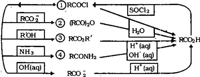
চিত্র ৯.৬ : কার্বক্সিলিক এসিডের জাতকসমূহের রূপান্তর তাগিকা
