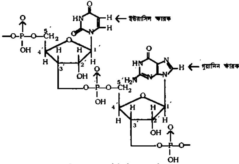
চিত্র ১১.২৩ : পলিনিউক্লিয়োটাইড শিকল।
