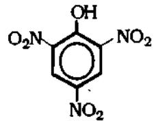
2,4,6-ট্রাইনাইট্রো ফেনল (পিকরিক এসিড)
