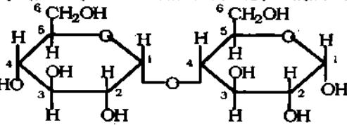
স্টার্চে \alpha -1, 4-গ্লাইকোসাইড বন্ধন
