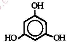
পিক্রিক এসিড বা 1,3,5-ট্রাইহাইড্রক্সি বেনজিন
