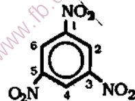
1,3,5-ট্রাই নাইট্রোবেনজিন
