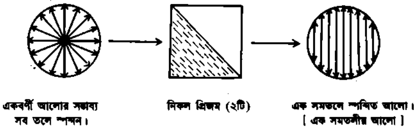
চিত্র ৪.১৭ : একবর্ণী আলোর বিভিন্ন তল, নিকল প্রিজম ও এক সমতলীয় আলো।
