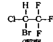
ফ্লোথেন 2-ব্রোমো-2-ক্লোরো-1, 1, 1- ট্রাইফ্লোরো ইথেন
