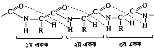
\alpha -হেলিক্স গঠনের প্রোটিন শিকল
