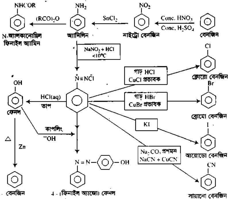
চিত্র ১০.৯ : ডায়াজেনিয়াম ক্লোরাইডের বিভিন্ন বিক্রিয়ার সর্বিৎসংসার
