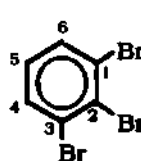
1,2,3-ট্রাইব্রোমো বেনজিন
