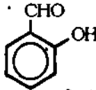
স্যালিসাইল অ্যালডিহাইড বা, 2-হাইড্রক্সি বেনজ্যালডিহাইড
