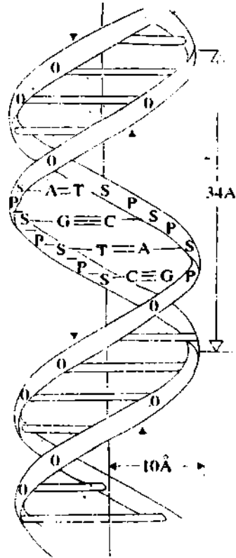
চিত্র ১১.২৫ : DNA এর জোড় কুণ্ডলী মডেল (বিহেলিক মডেল)। (..... হাইড্রোজেন বন্ধন)।
