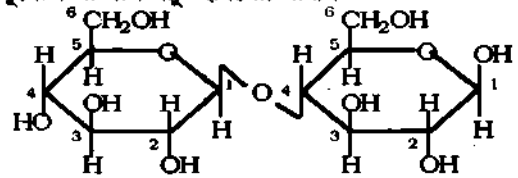
সেলুলোজে \beta -1, 4- গ্লাইকোসাইড বন্ধন
