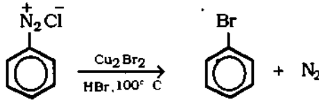
ব্রোমোবেনজিন
