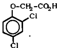
2, 4-D
