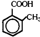
অর্ধে টলুয়িক এসিড বা 2-মিথাইল বেনজোয়িক এসিড
