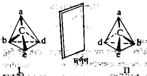
চিত্র ৪.২০ : Cabde অণুর চতুস্তলকীয় গঠন ও এর দর্পণ প্রতিবিম্ব।
