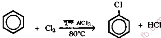
ক্লোরো বেনজিন
