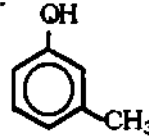
মটা ক্রিসল বা 3-মিথাইল ফেনল
