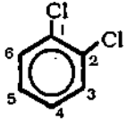
1, 2.-ডাইক্লোরো বেনজিন
