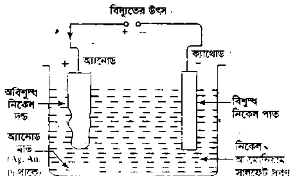
চিত্র ৩.১৩ : অশিশু নিকেলের বিদ্যুৎ বিশুদ্ধীকরণ।
